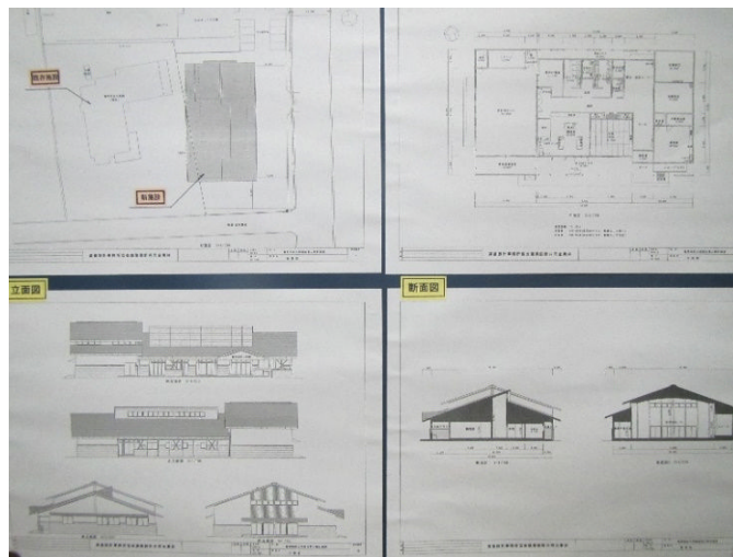
配置図、平面図、立面図、断面図を掲示しています
