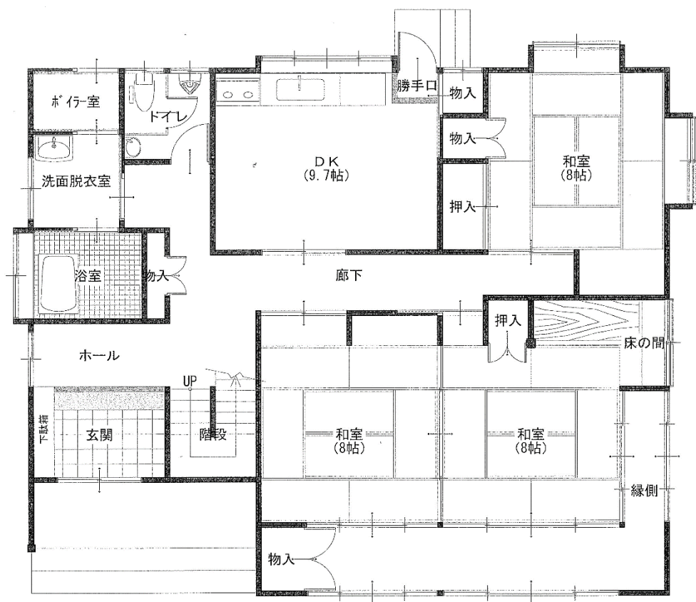
1階 平面図 S:1/65
